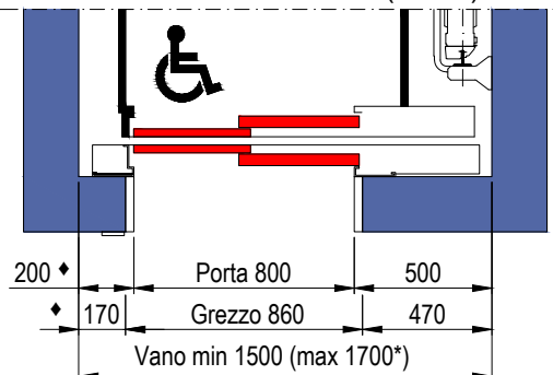
PIANTA VANO CORSA PORTE SENZA TELAI (EI120)
