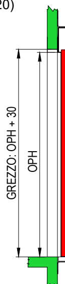
SEZIONE PORTE SENZA TELAIO (EI120)
